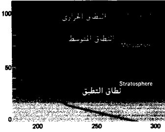
شكل (138) يوضح التغير في درجة الحرارة مع الارتفاع في الغلاف الغازي للأرض
